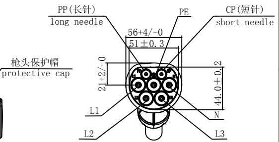
16A桩端插头7POS 16A pile end plug 7POS
